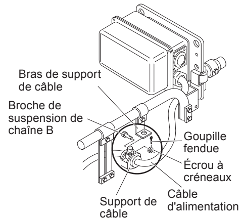
<Cordon de l'interrupteur à bouton-poussoir pour 15 t à 20 t> <Connexion du câble d'alimentation du chariot>
