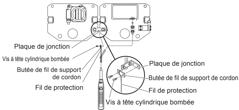
<Cordon de l'interrupteur à bouton-poussoir pour 15 t à 20 t> <Connexion du câble d'alimentation du chariot>
