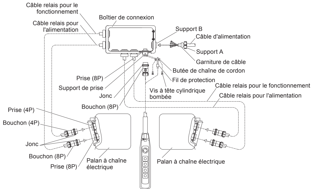
<Cordon de l'interrupteur à bouton-poussoir pour 15 t à 20 t> <Connexion du câble d'alimentation du chariot>
