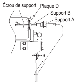
<Connexion du cordon de l'interrupteur à bouton-poussoir à montage direct>
